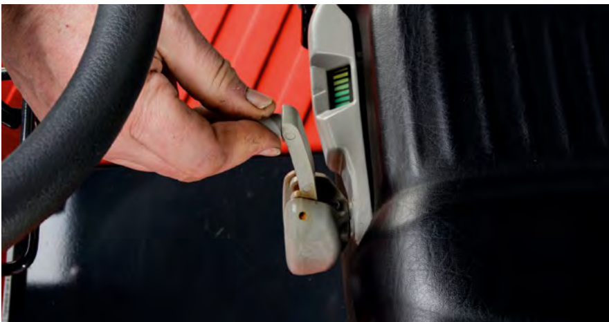
gewichtsabhängige Sitzeinstellung
